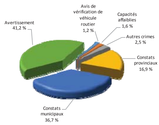
Graphique 4 : Catégories d'interventions
